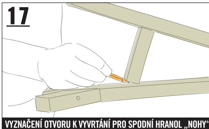
PŘEDVRTÁNÍ
