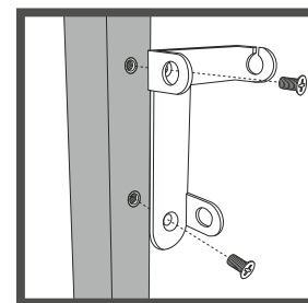
HORNÍ UZAMČENÍ BRÁNY
