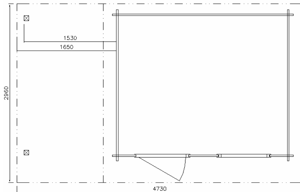
PŮDORYS
