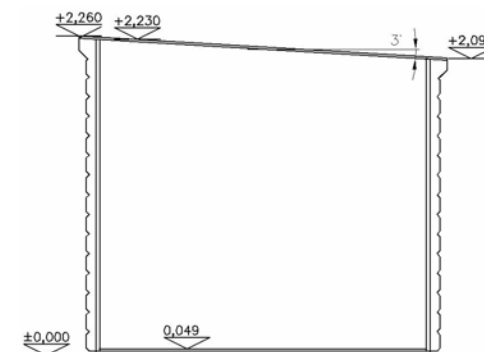
ŘEZ
