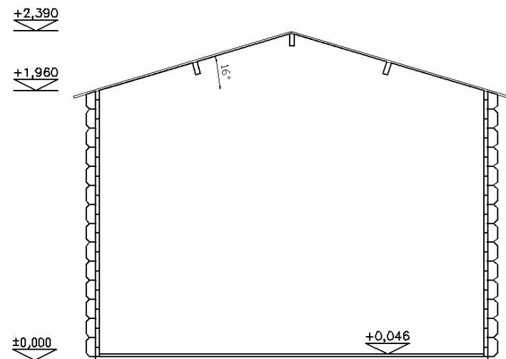
ŘEZ
