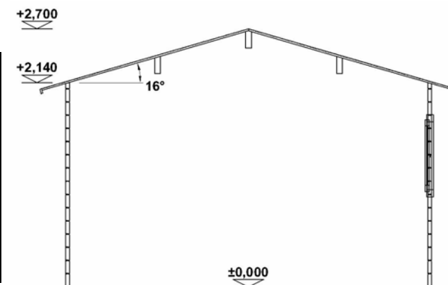
ŘEZ
