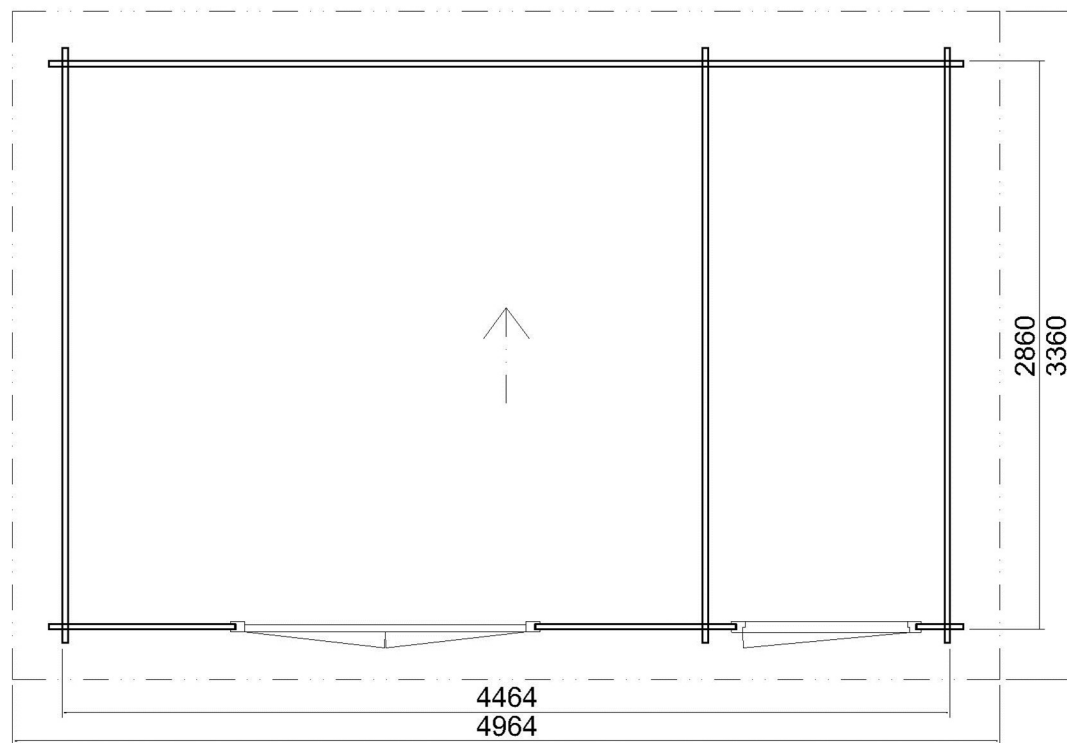
PŮDORYS
