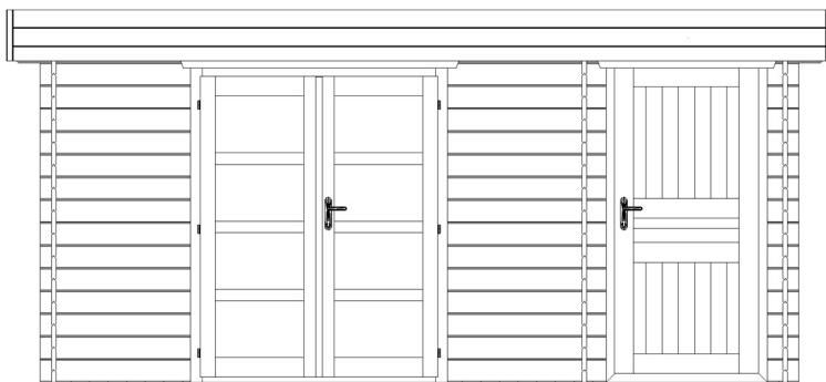
PŘEDNÍ POHLED
