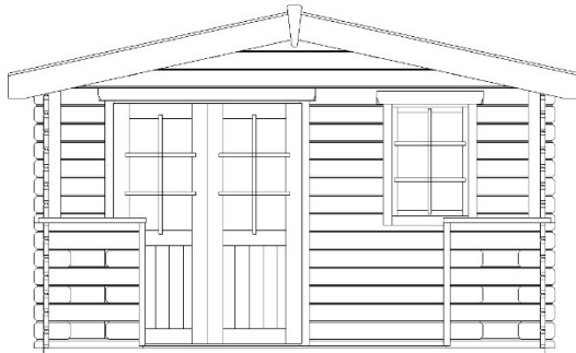
PŘEDNÍ POHLED
