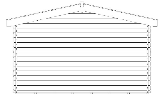
ZADNÍ POHLED
