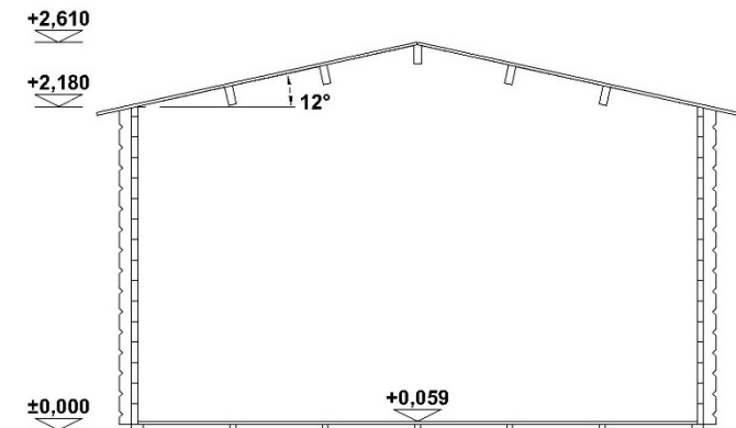
ŘEZ
