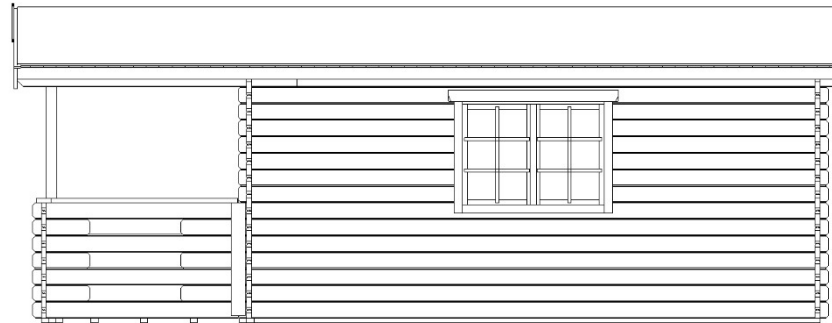
BOČNÍ POHLED PRAVÝ
