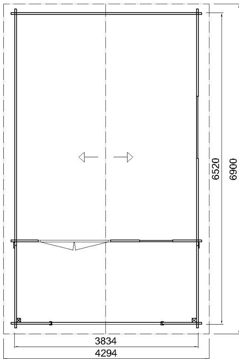
PŮDORYS
