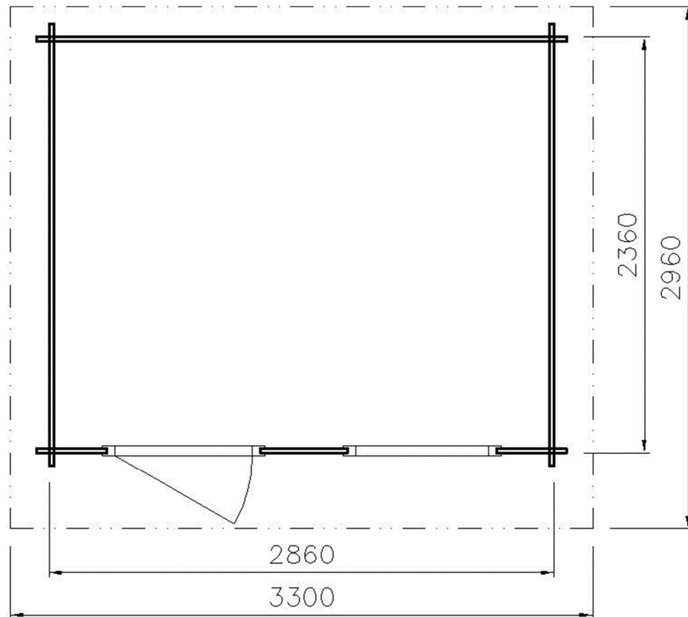
PŮDORYS
