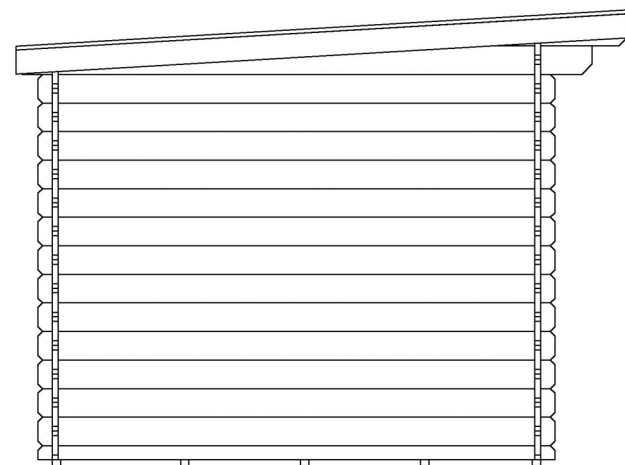
BOČNÍ POHLED LEVÝ
