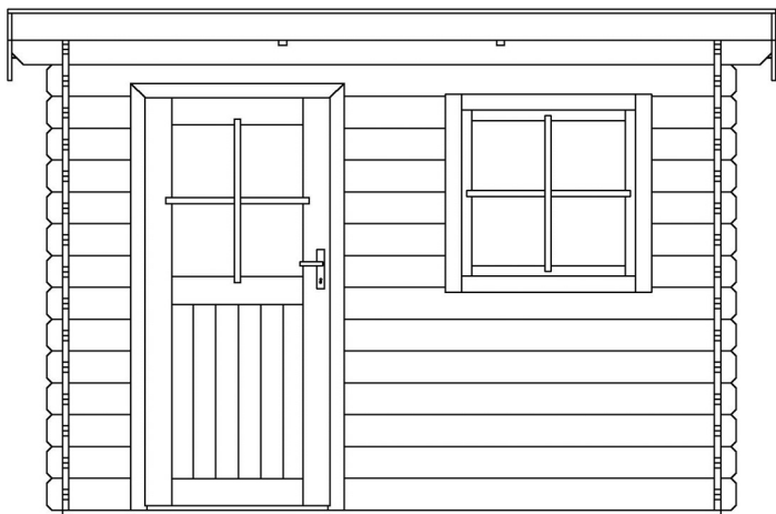
PŘEDNÍ POHLED
