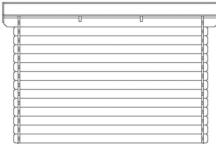
ZADNÍ POHLED
