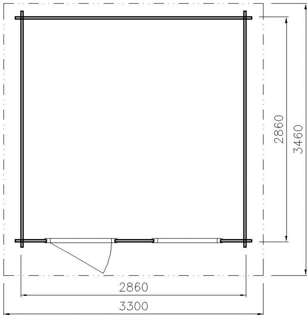
PŮDORYS
