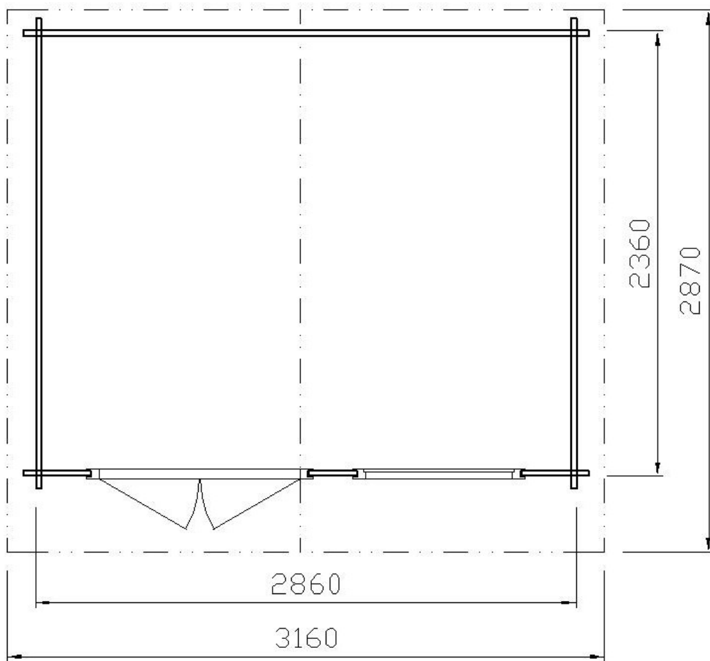
PŮDORYS
