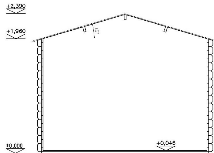
ŘEZ
