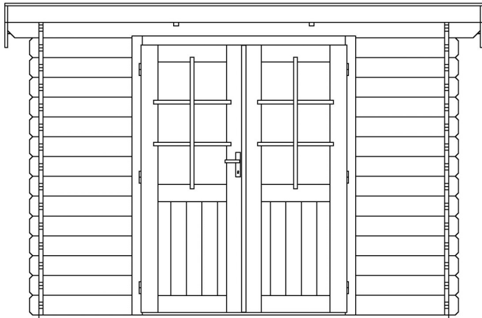
PŘEDNÍ POHLED
