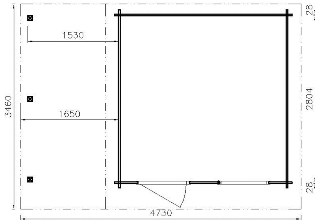
PŮDORYS
