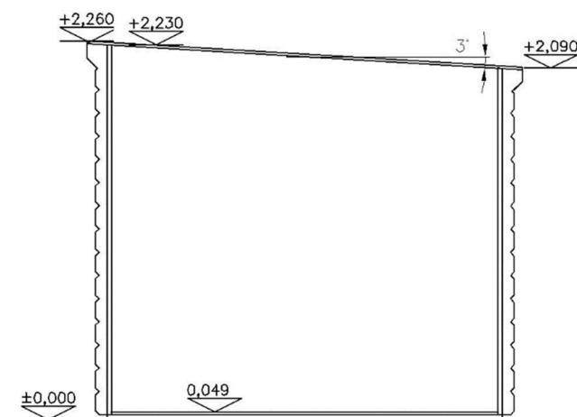
ŘEZ
