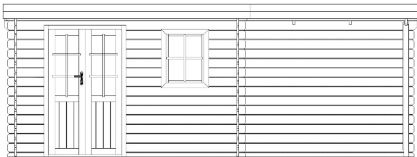
PŘEDNÍ POHLED
