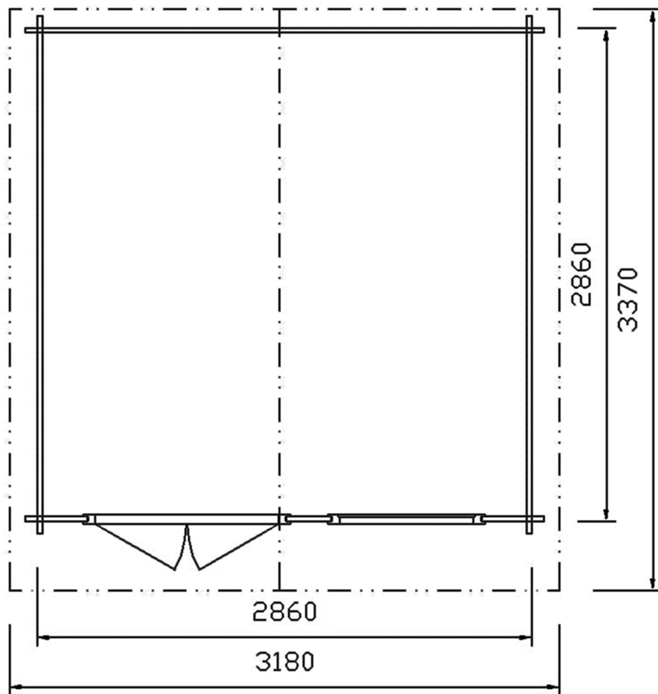
PŮDORYS
