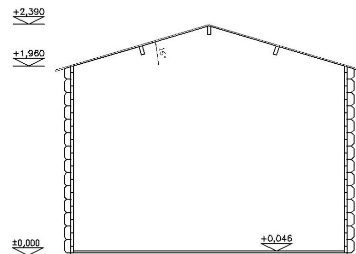
ŘEZ
