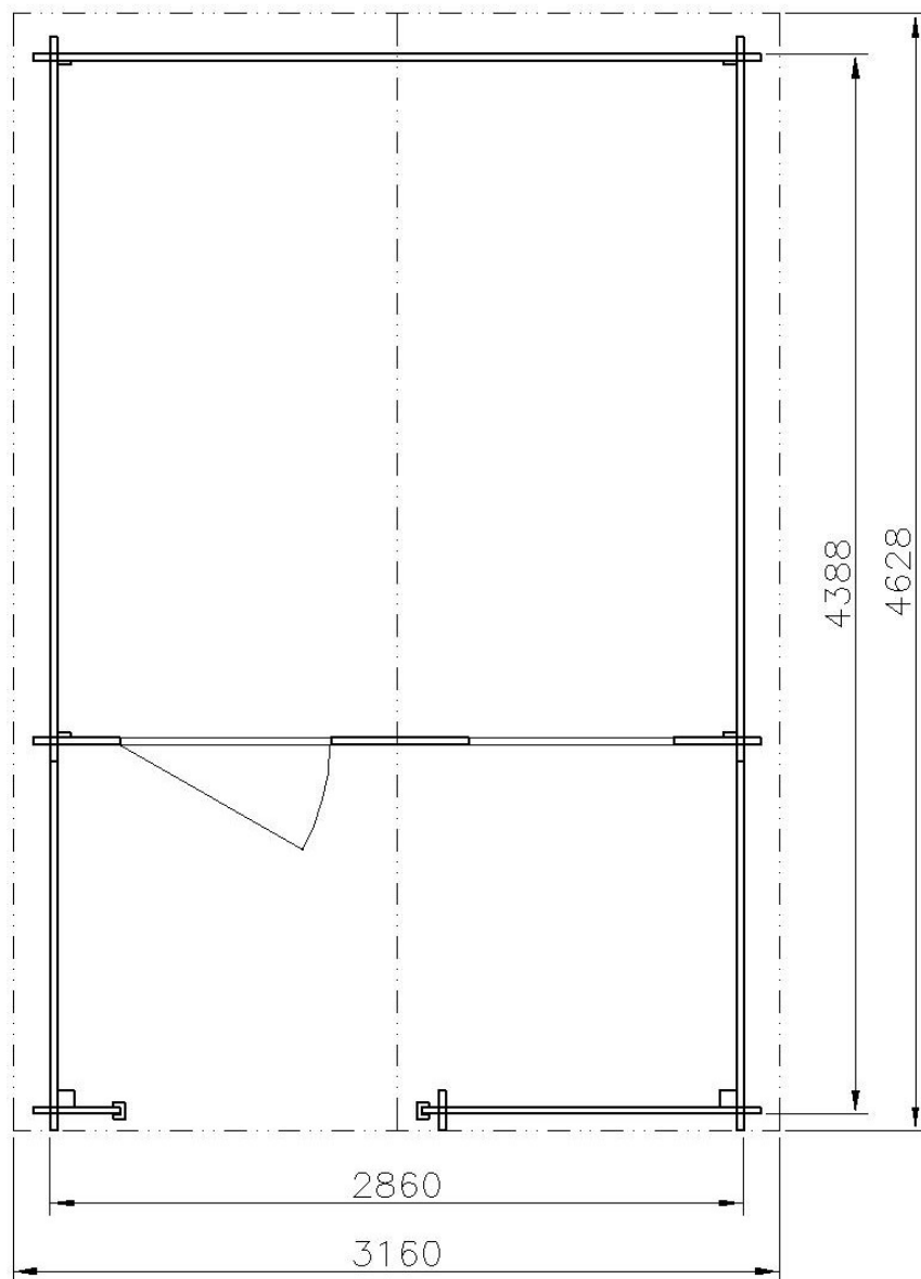
PŮDORYS
