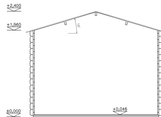
ŘEZ
