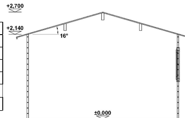
ŘEZ
