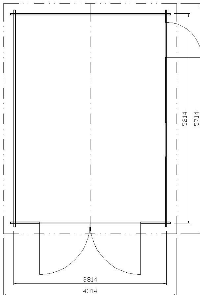
PŮDORYS
