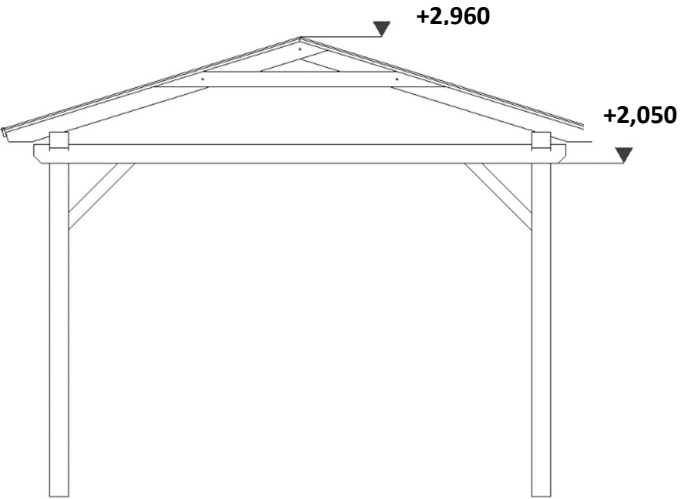
ŘEZ
