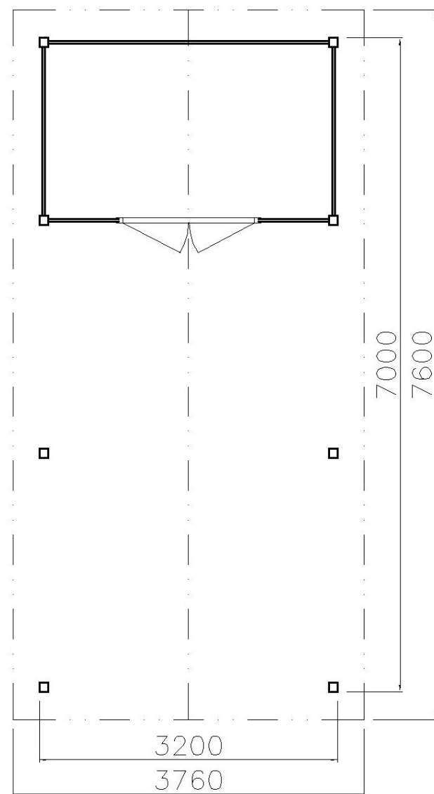
PŮDORYS
