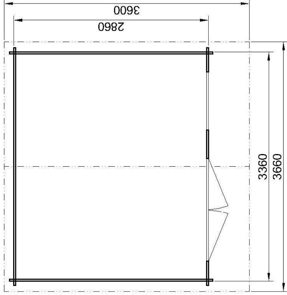
PŮDORYS
