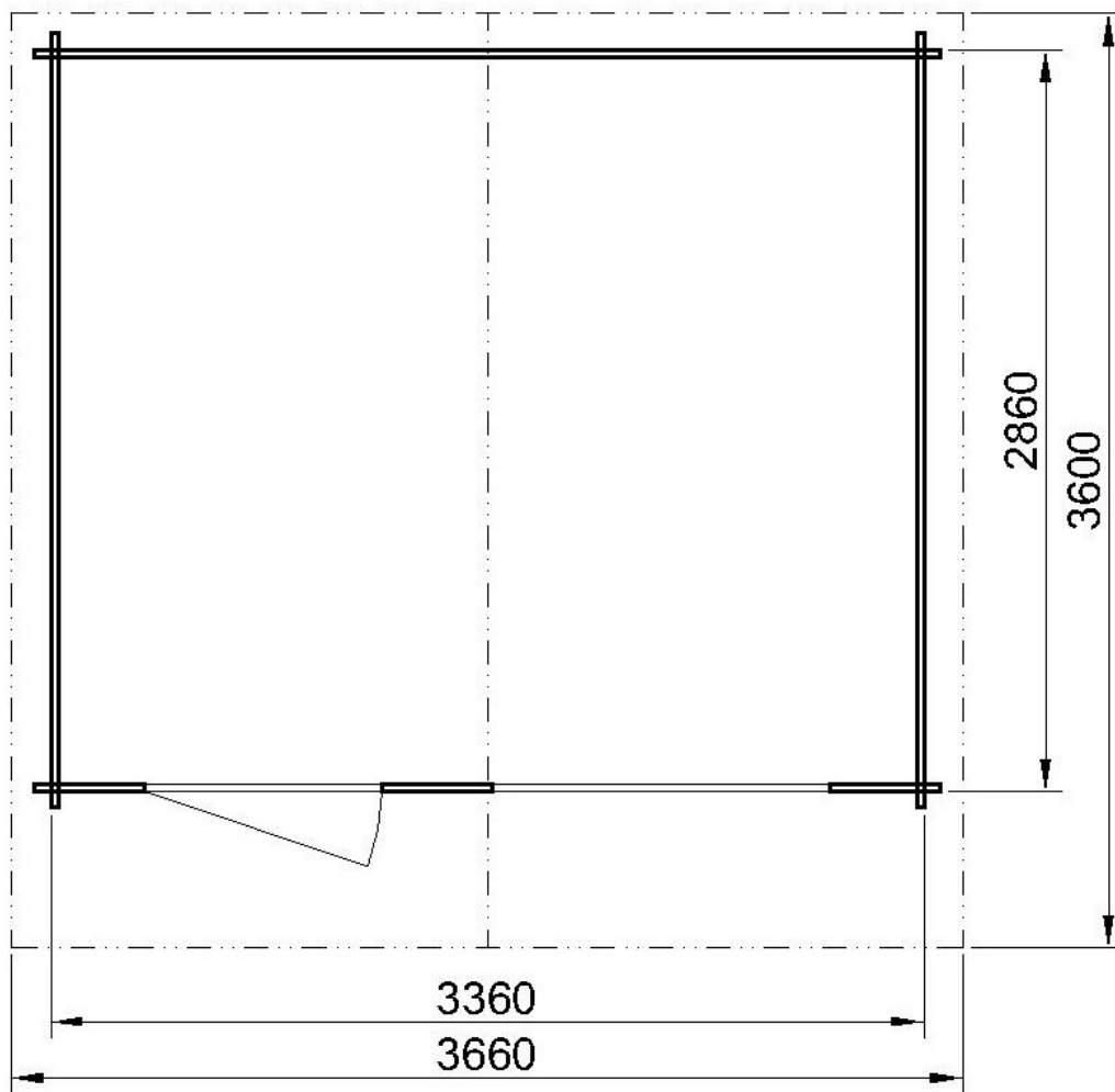
PŮDORYS
