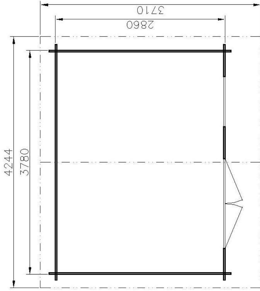
PŮDORYS
