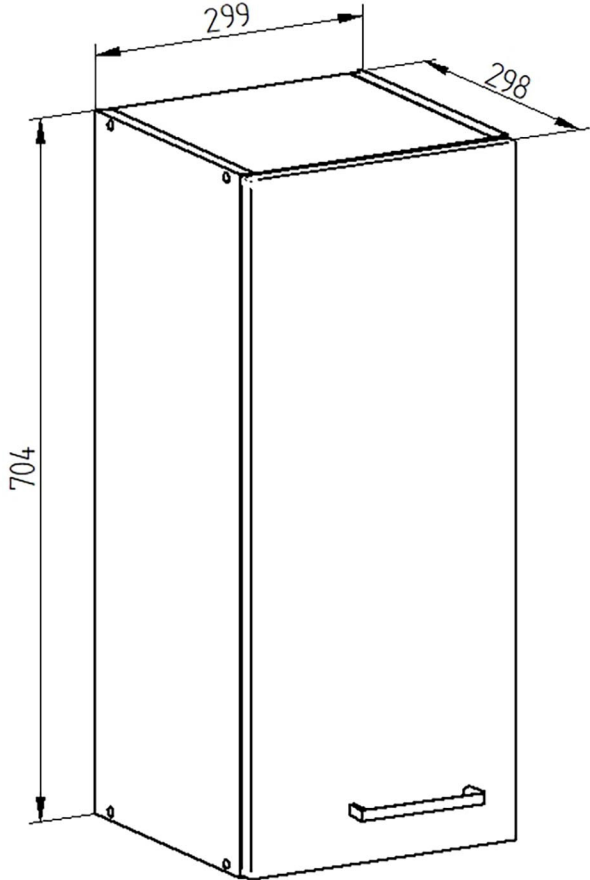
TYP H 30
