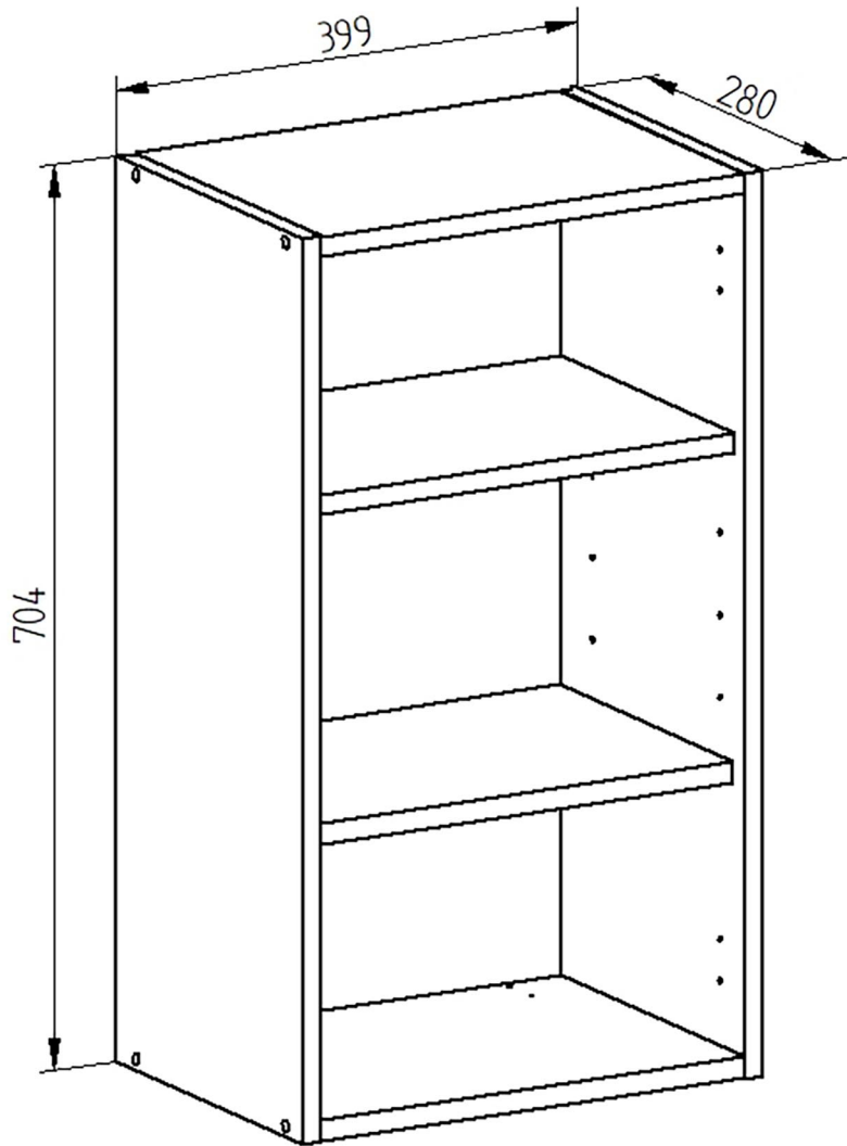
TYP H 40
