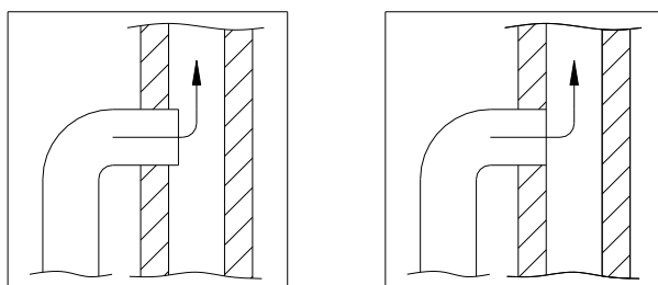
obr. č.1 Připojení na komín
