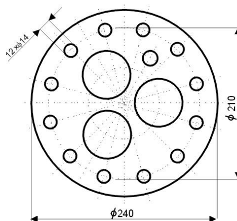
Uchycení 12 x M12
