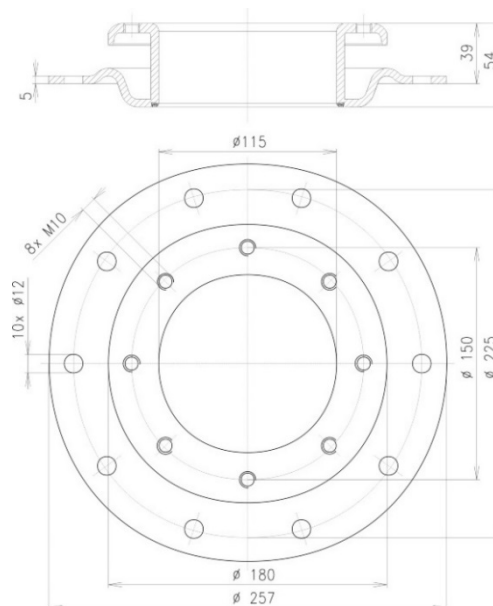
Redukční příruba 225 / 150
