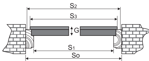
WIDOK PIONOWY DRZWI / AJTÓ FÜGGŐLEGES METSZET / VERTIKÁLNI POHLED / VERTIKÁLNI POHLED / VERTICAL VIEW OF THE DOOR / VEDERE - UȘĂ VERTICALĂ / VUE VERTICALE DE LA PORTE
