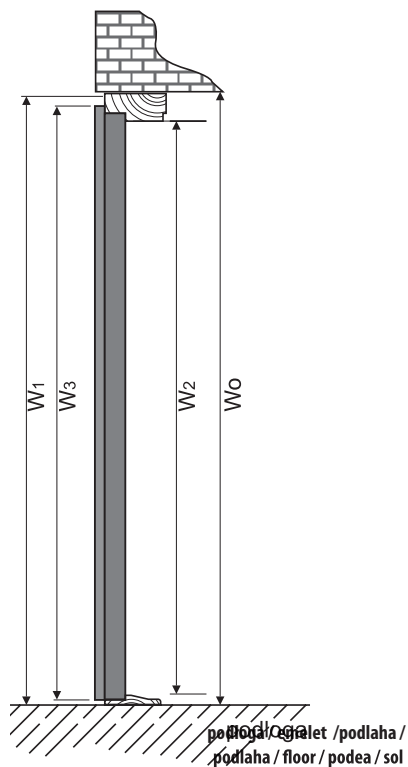
WIDOK POZIOMY DRZWI / AJTÓ VÍZSZINTES METSZET / HORIZONTALNY POHLED / HORIZONTALNY POHLED / HORIZONTAL VIEW OF THE DOOR / VEDERE - NIVEL UȘĂ / VUE HORIZONTALE DE LA PORTE
