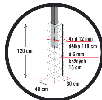
VYZTUŽENÍ ZÁKLADŮ SLOUPKŮ
