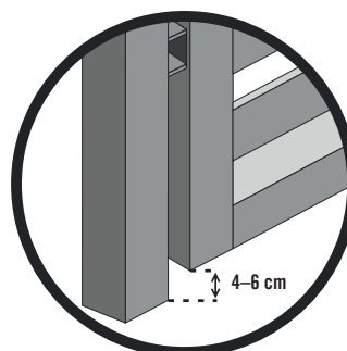
VZDÁLENOST KŘÍDLA BRÁNY A BRANKY OD POVRCHU
