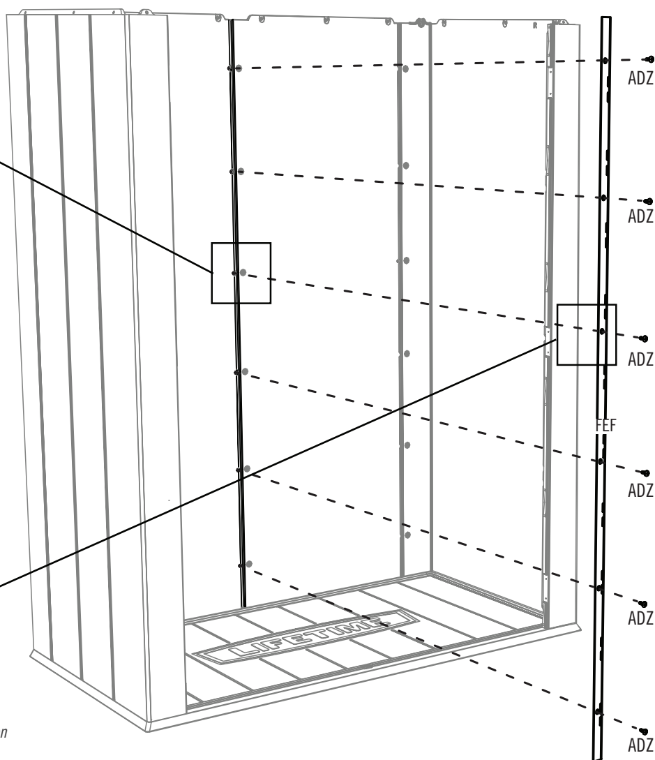
Foro nel canale / Loch im Profil / Отверстие в швеллере
