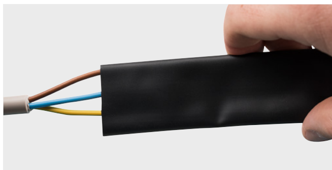
Navlečte smršťovací bužíрку.
