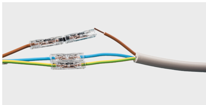
Nasadte svorku a přetáhněte smršťovací bužíрку.
