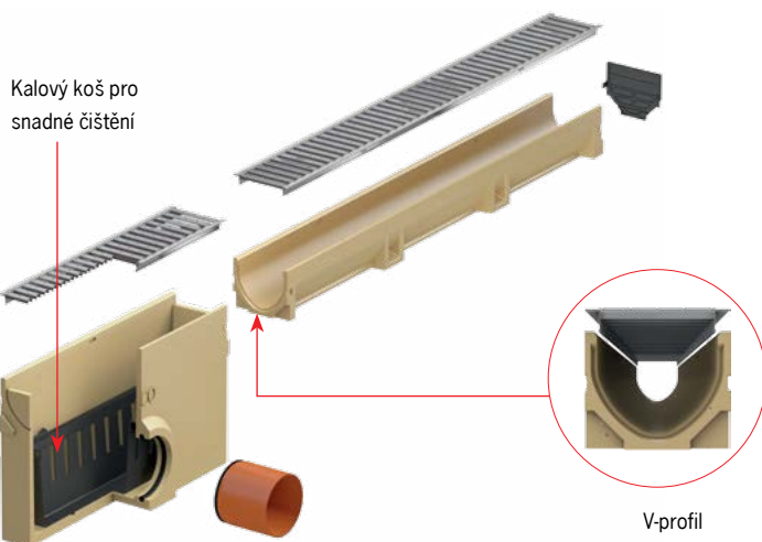
Odtok ze žlabu a napojení na potrubí pomocí systémové vpusti
