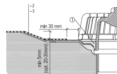
3.2.a Detail napojení folie mPVC (TPO-FPO)
