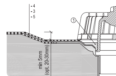
3.2.b Detail napojení folie z asfaltových pásů
