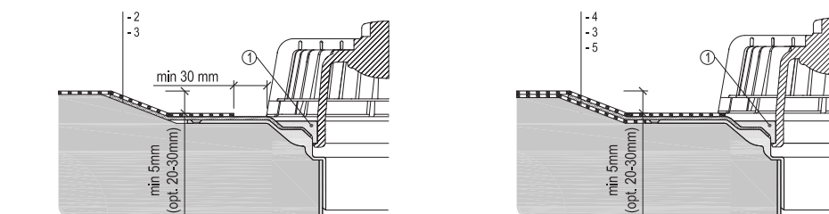
3.2.a a lágy PVC (TPO-FPO) fólia csatlakoztatásának részlete
