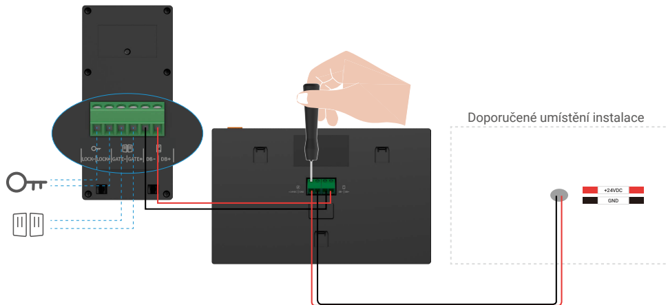
1-1 Schéma zapojení
