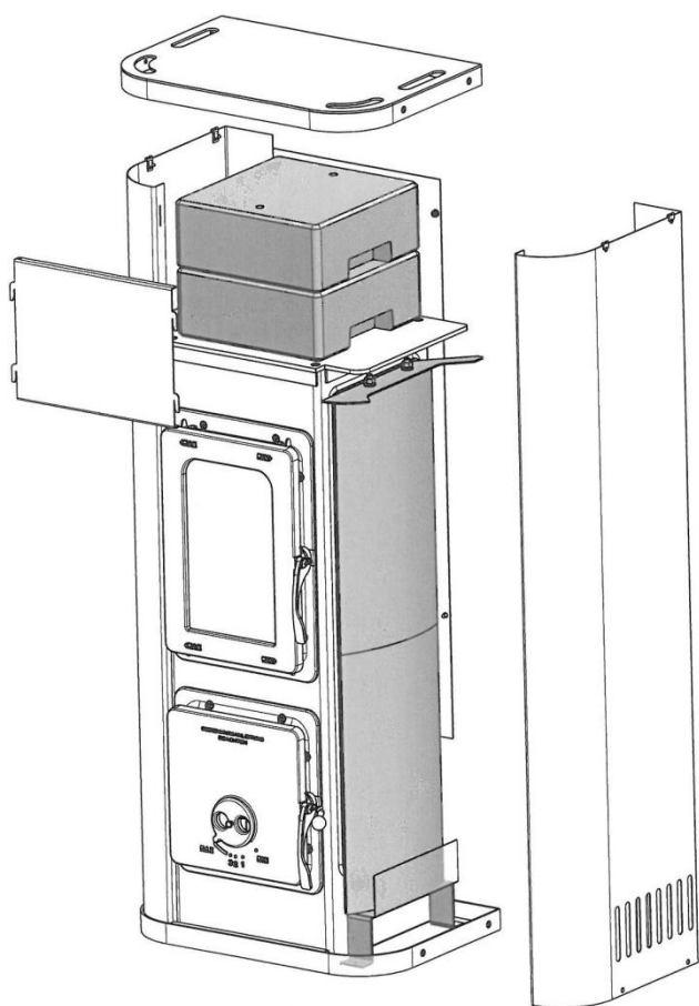
BRIXEN + AK
