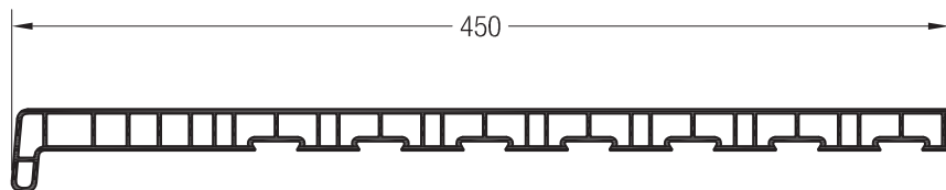
Vnitřní parapet 450
