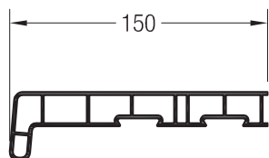
Vnitřní parapet 150
