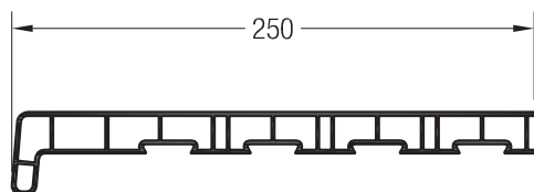
Vnitřní parapet 250
