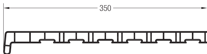
Vnitřní parapet 350
