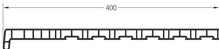
Vnitřní parapet 400
