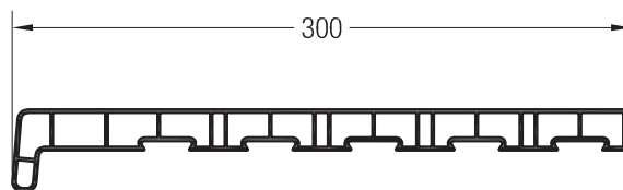
Vnitřní parapet 300
