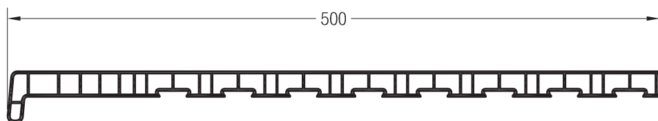
Vnitřní parapet 500
