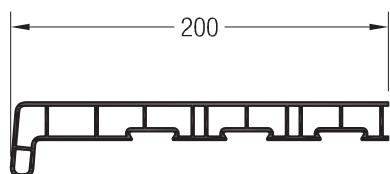
Vnitřní parapet 200
