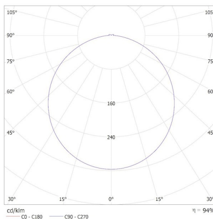
KANLUX S.A. (kat 26779) AVAR 6060 32W-CCT / Krzywa rozsyłu światła (biegunowo)
