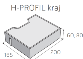
H-PROFIL kraj tl. 6cm
