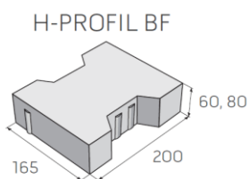
H-PROFIL skladba tl. 6cm
