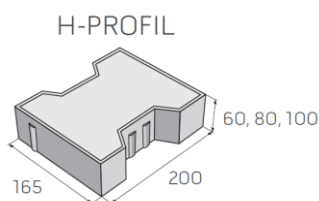
H-PROFIL tl. 6cm
