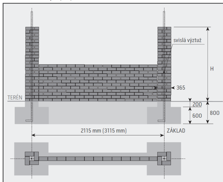
Schéma osazení sloupků (mm)
