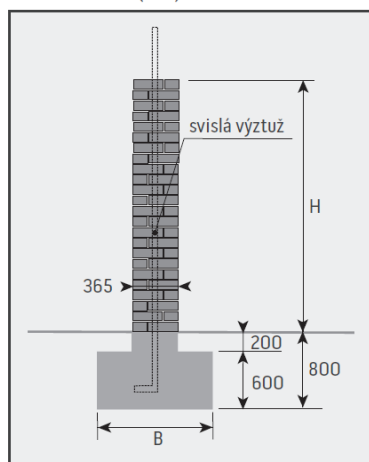
Schéma základu (mm)
