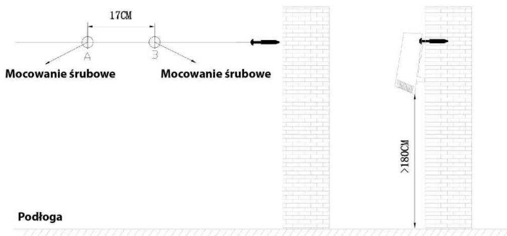
Rysunki instalacyjne: montaż na ścianie
